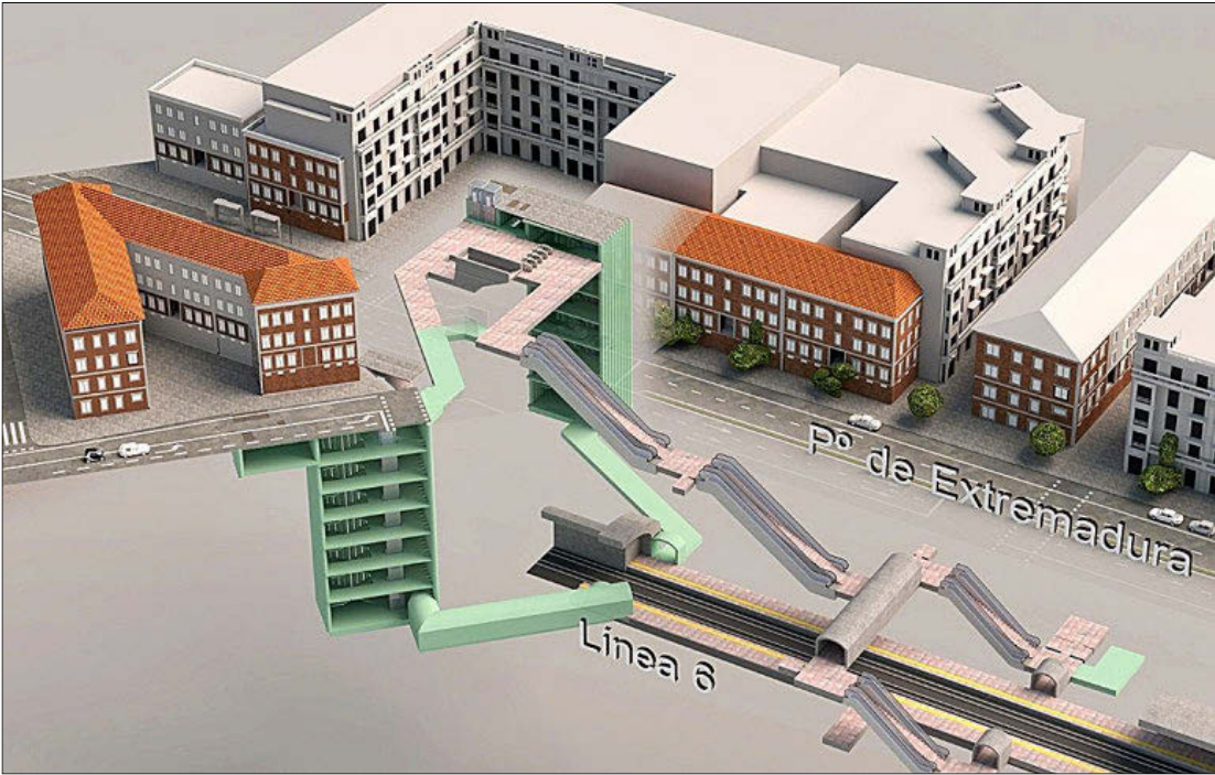
Infografía de la instalación de nuevos ascensores en la estación de Metro de Alto de Extremadura. METRO DE MADRID
